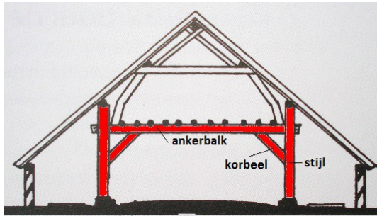
Het ankerbalkgebint in dwarsdoorsnede
