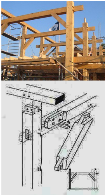
Het ankerbalkgebint op de foto en op een ontwerptekening
